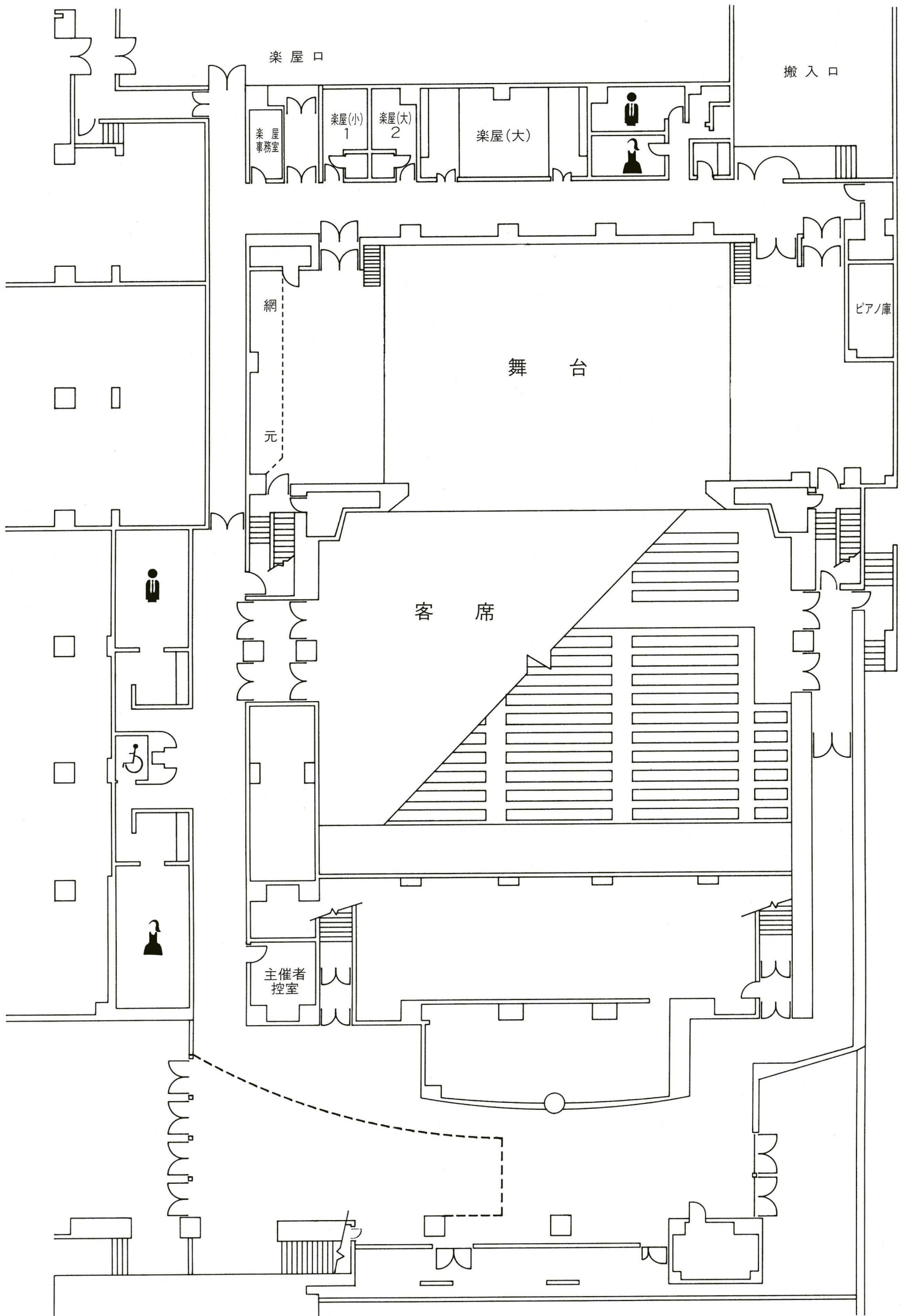
文化会館棟一階平面図(1/200)
